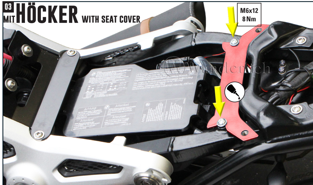
03 MIT HÖCKER WITH SEAT COVER Paßt auch mit 31742-3xx. Also fits with 31742-3xx.
