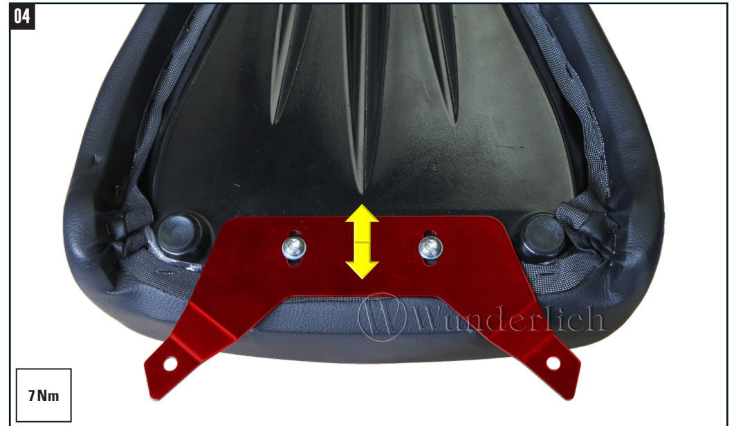
04 Halter so ausrichten, das sich Höcker oder Beifahrersitz spannungsfrei montieren lassen. Adjust the bracket until the hump or passenger seat can be mounted free of strain.
